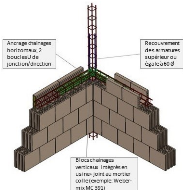
Figure 20 Détail jonction angle blocs chainages verticaux intégrés en usine (toutes zones sismiques)
