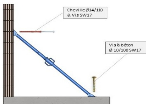
Figure 1 : Etais tirant poussant
