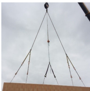
Figure 6 : Equilibrage des élingues par poulies
