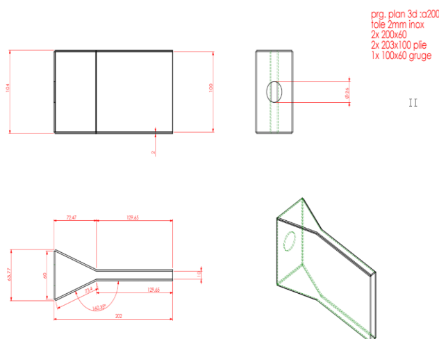
Figure 32 Dimensions "bec" de collage des joints verticaux
