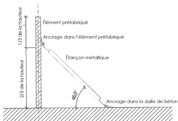
Figure 17 - Pose des étais tirant poussant et des renforcements lors d'une pose sur support béton armé
