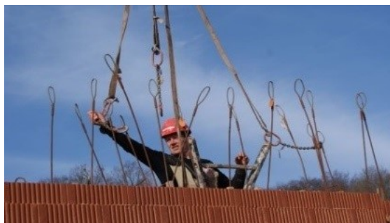
Figure 9 Boucles de levage
