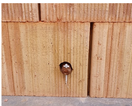
Figure 11 Broche d'ancrage en pied de mur
