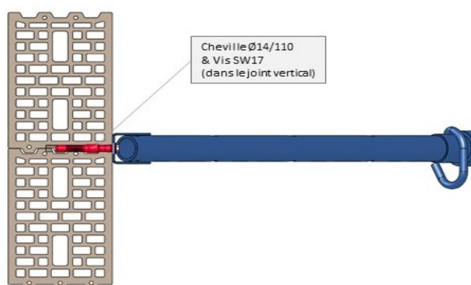
Figure 2 : Chevilles d'ancrage
