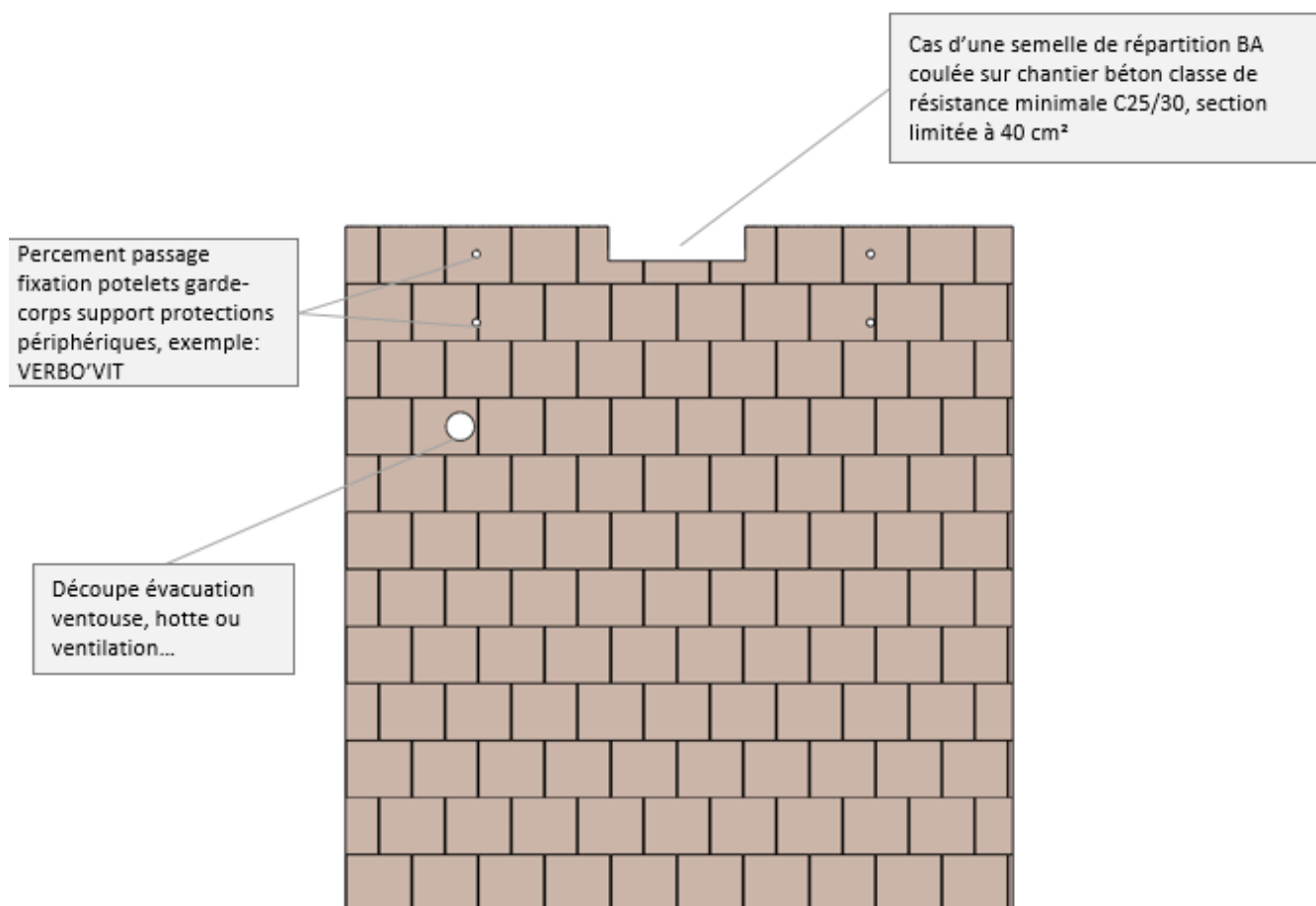
Figure 34 Détail option réservations sur mesures en usine dans les MUR TERRE CUITE PREFAXIS
